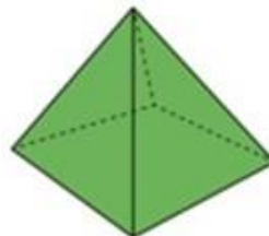
Une pyramide
