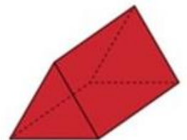
Un prisme
